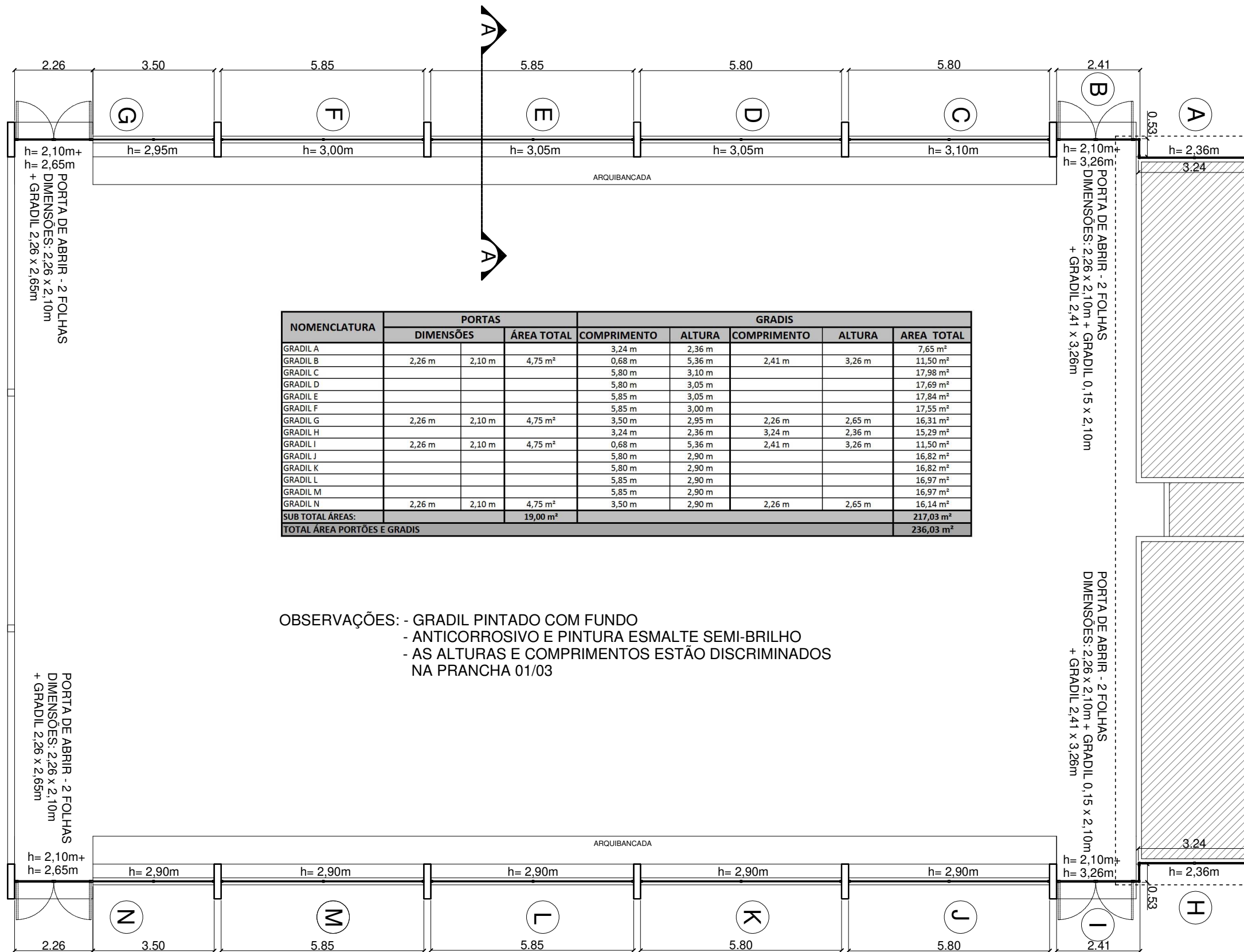
PLANTA DE LOCALIZAÇÃO DOS GRADIS Esc.: 1/125
